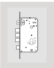
9 Замок
